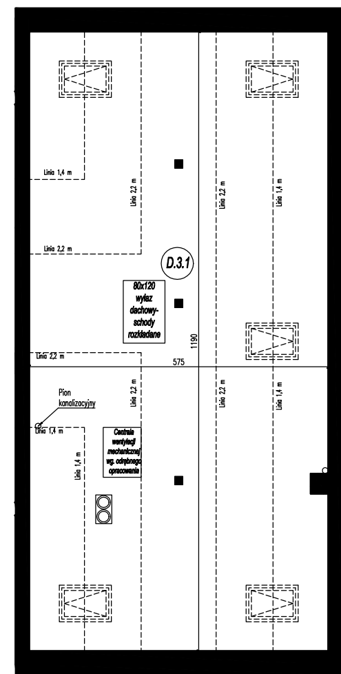
LOKAL D- powierzchnie poddasze Nr. Pom. Nazwa Pom. Pow. m2 D.3.1 Poddasze nieużytkowe 34,40
