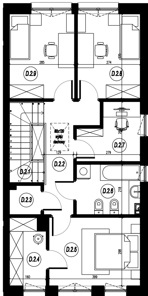
LOKAL D- powierzchnie piętro Nr. Pom. Nazwa Pom. Pow. m2 D.2.1 Schody 4,54 D.2.2 Korytarz 7,55 D.2.3 Magazynek 1,60 D.2.4 Garderoba 4,50 D.2.5 Sypialnia 1 11,89 D.2.6 Łazienka 6,00 D.2.7 Gabinet 5,90 D.2.8 Sypialnia 2 10,10 D.2.9 Sypialnia 3 10,50
