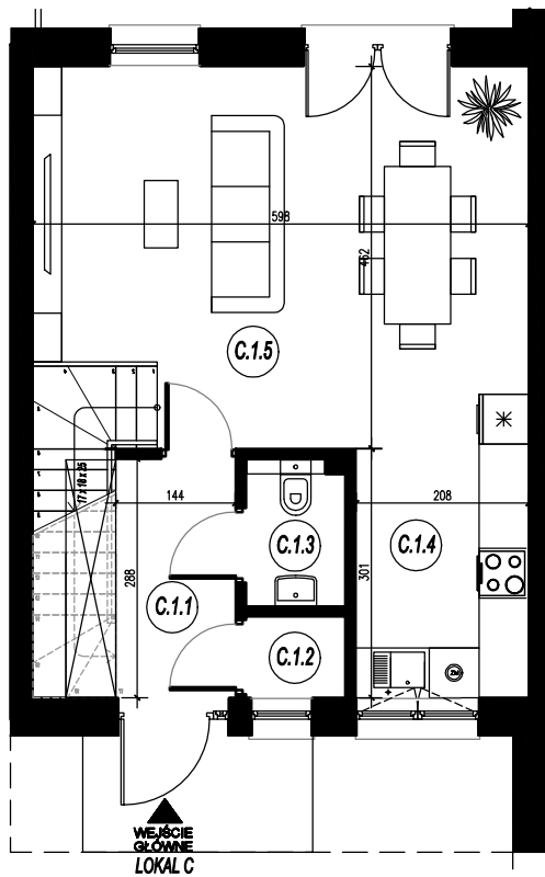
1 RZUT PARTERU
