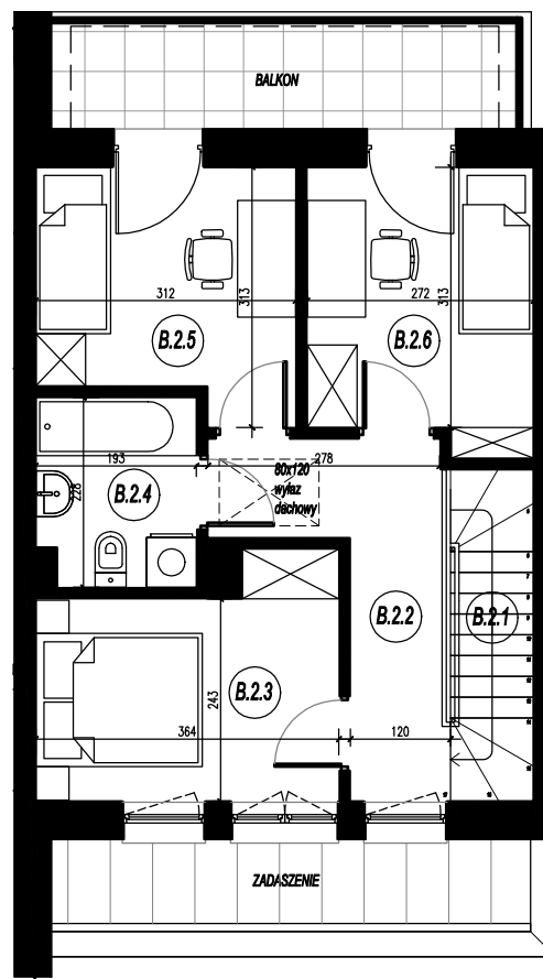
2 RZUT PIĘTRA
