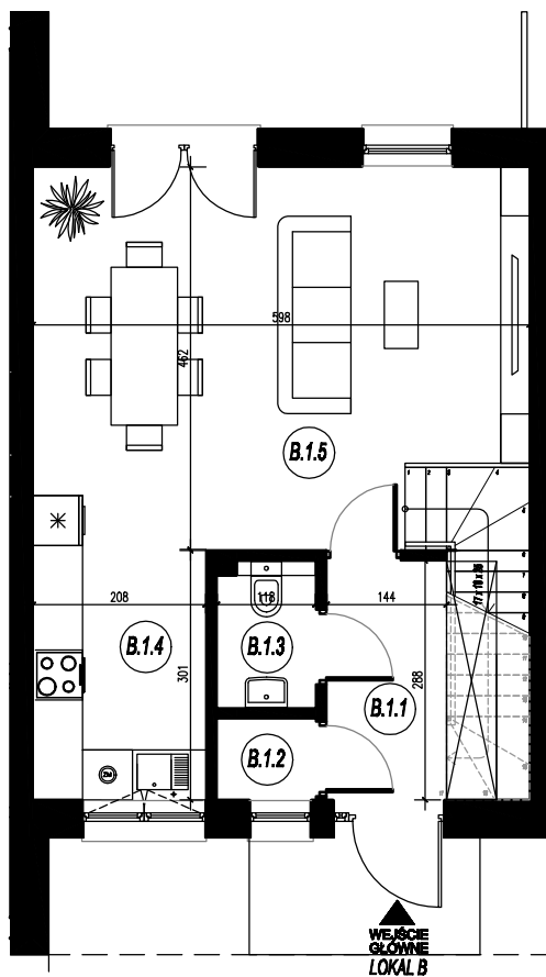
1 RZUT PARTERU
