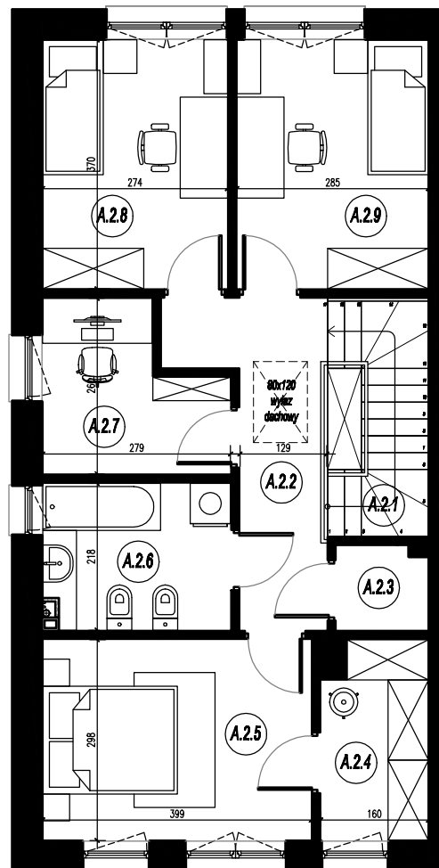
2 RZUT PIĘTRA
