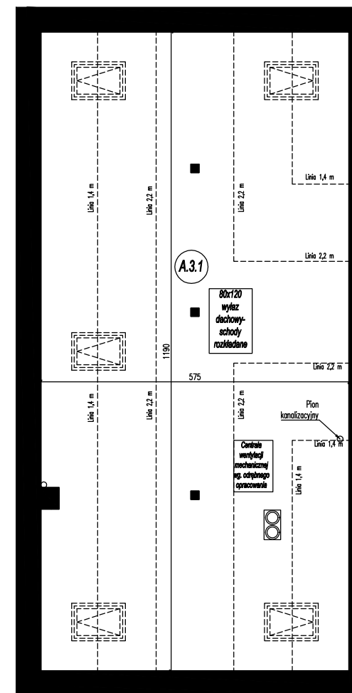
3 PODDASZE
